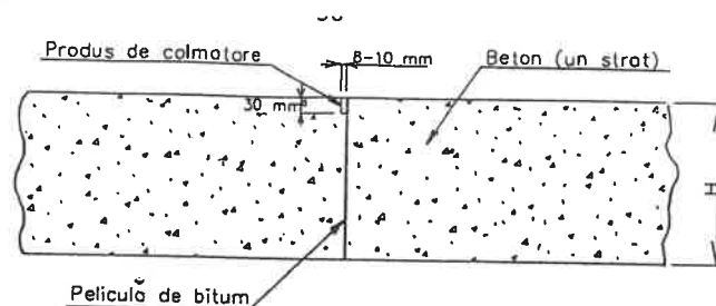
Fig. 9 Rost de contact transversal la îmbrăcăminți executate într-un strat
