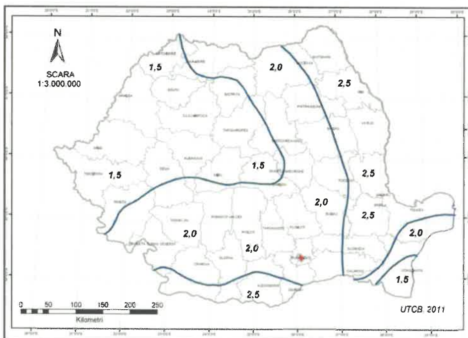
Fig.4. Încărcarea din zăpadă pe sol S_z
