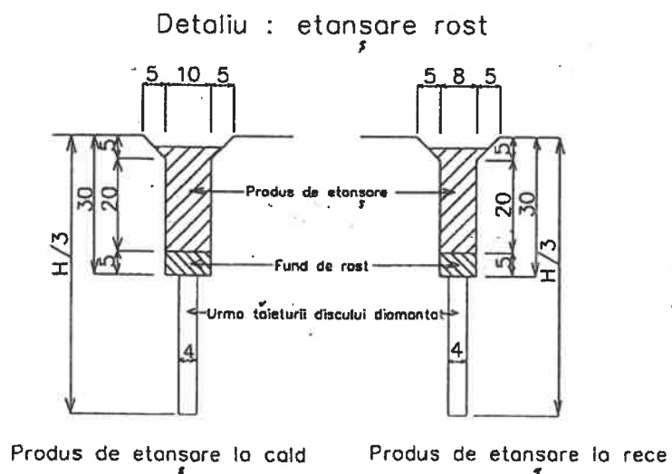
Fig. 19 Rost transversal de contractie, executat pe toată lățimea îmbrăcăminte
