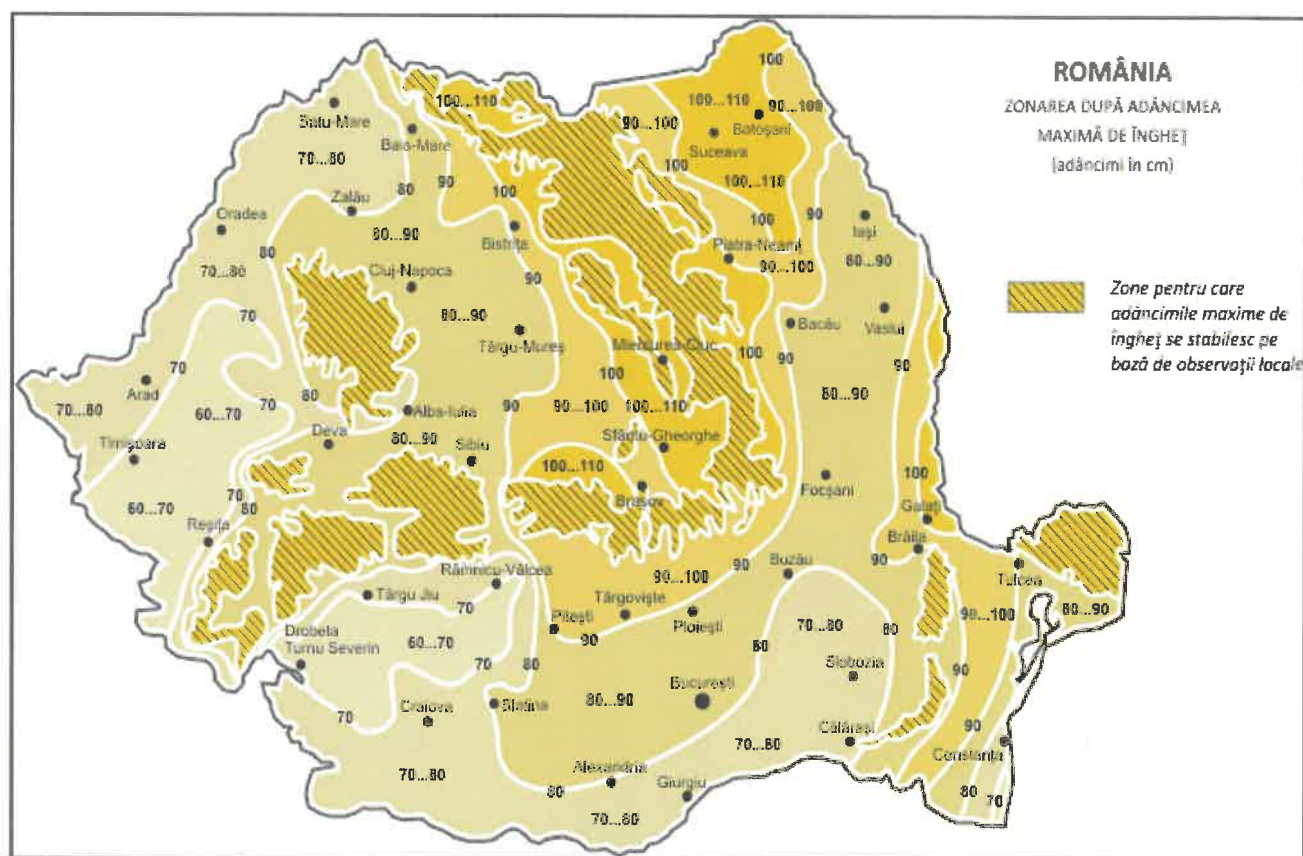
Fig.2. Zonarea după adâncimea de îngheț
