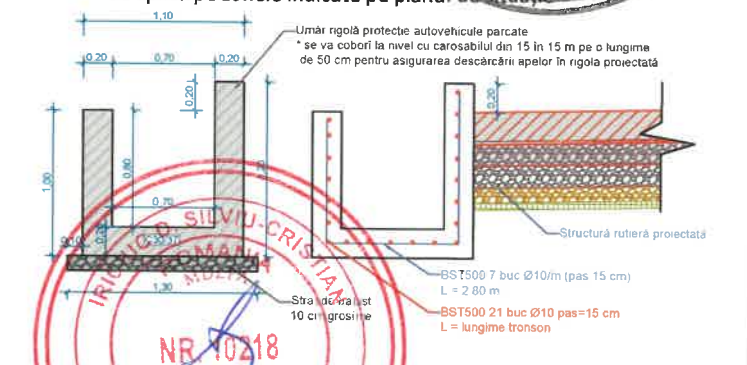
Detaliu rigolă din beton armat
