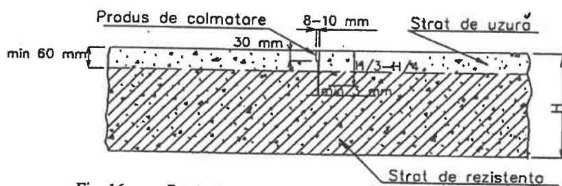
Fig. 16a Rost de contracție transversal, la imbrăcăminti în două straturi, executate cu două discuri diferite
