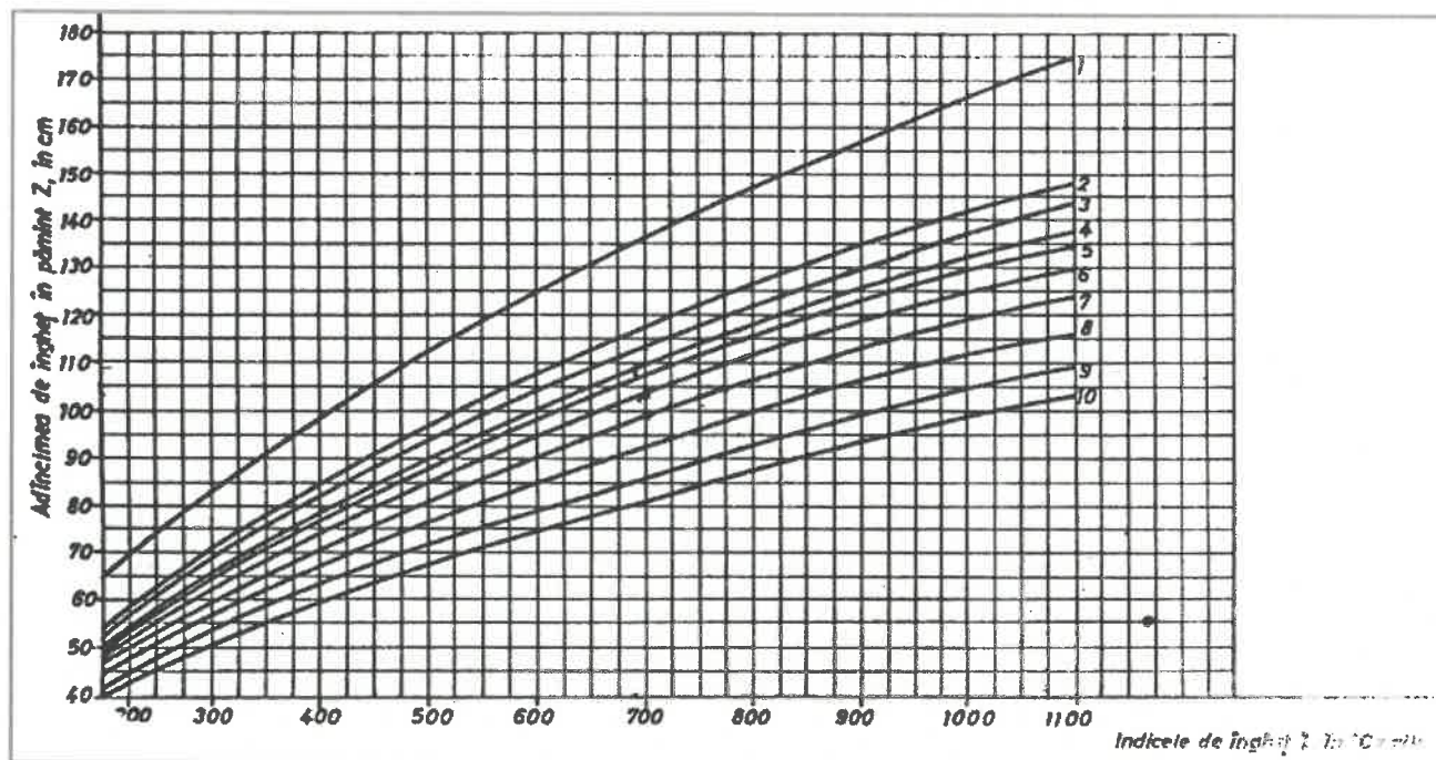
Fig. 2 – Adâncimea de îngheț
