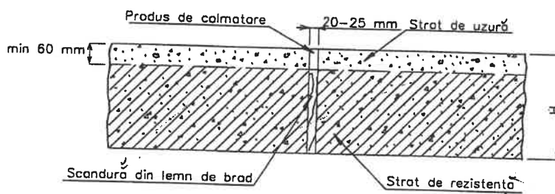
Fig. 14 Rost de dilatație transversal, la îmbrăcămîni executate în două straturi
