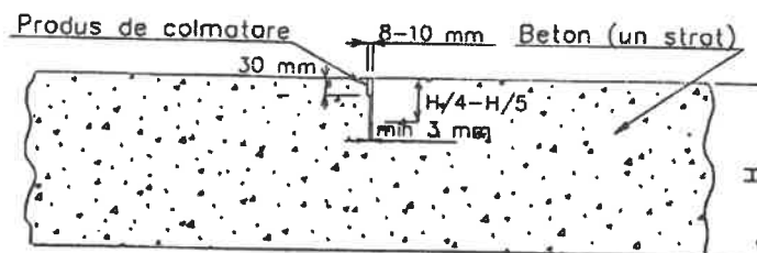
Fig. 15a Rost de contracție transversal, la imbrăcăminti într-un strat, executate cu două discuri diferite
