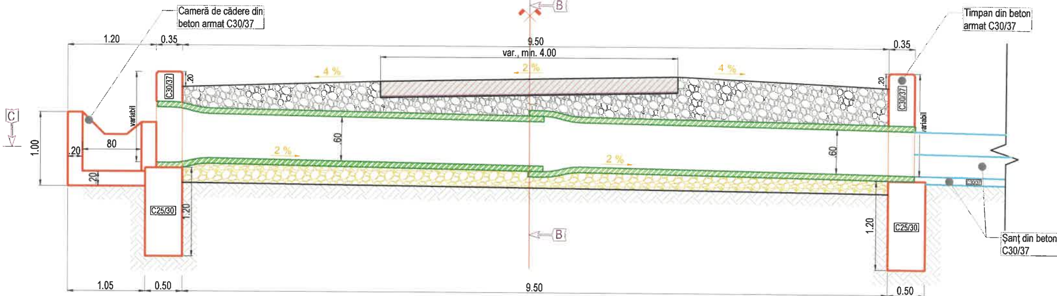
SECȚIUNE LONGITUDINALĂ A-A scara 1:50
