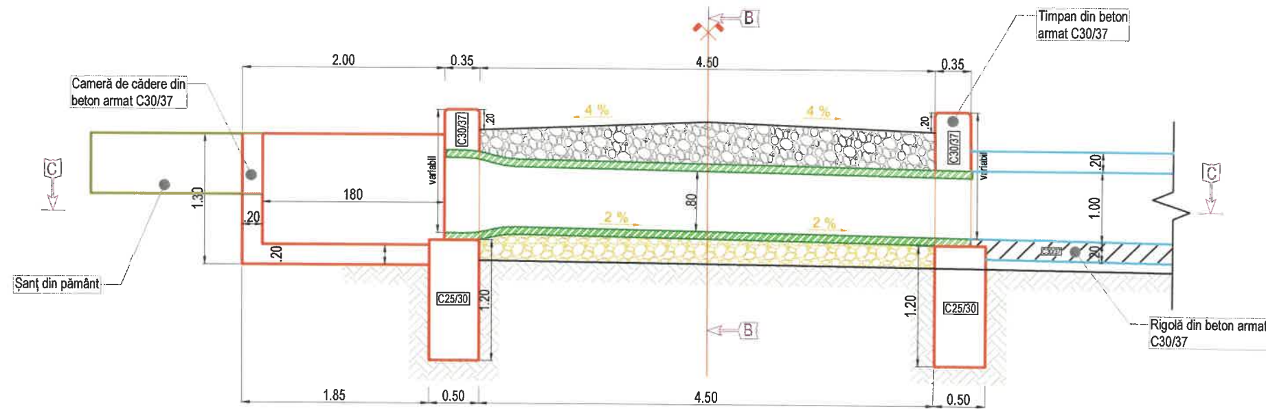
SECȚIUNE LONGITUDINALĂ A-A
