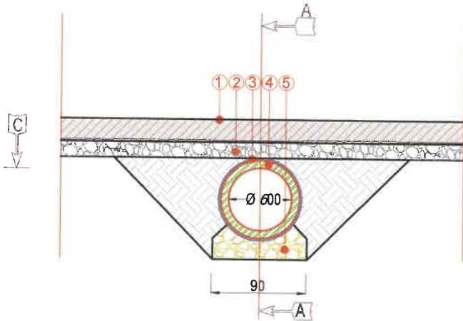
SECȚIUNE TRANSVERSALĂ B-B scara 1:50
