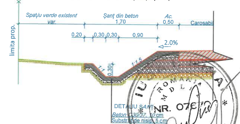
Detaliu rigolă din beton armat
