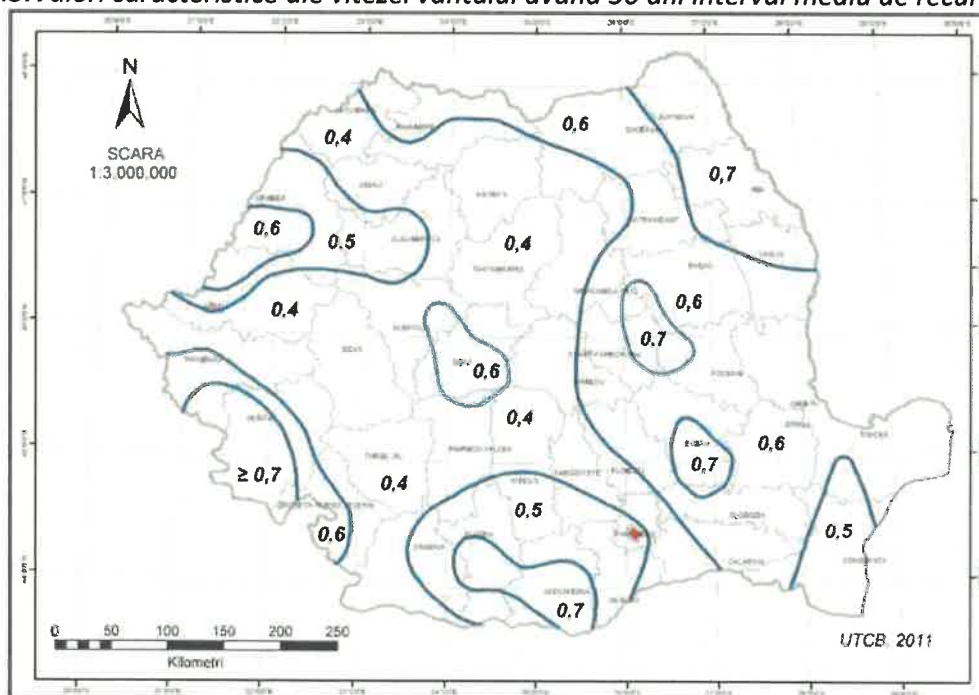
Fig.6.Valori caracteristice ale presiunii de referință a vântului, mediata pe 10 min.
