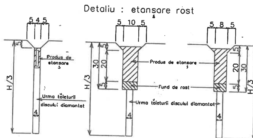
Fig. 17 Rost longitudinal de contracție la benzi cu lățimea mai mare de 5.00 m
