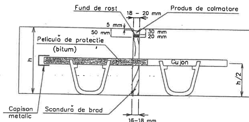
Fig. 22 – Detaliu, rost de dilatație gujonat
