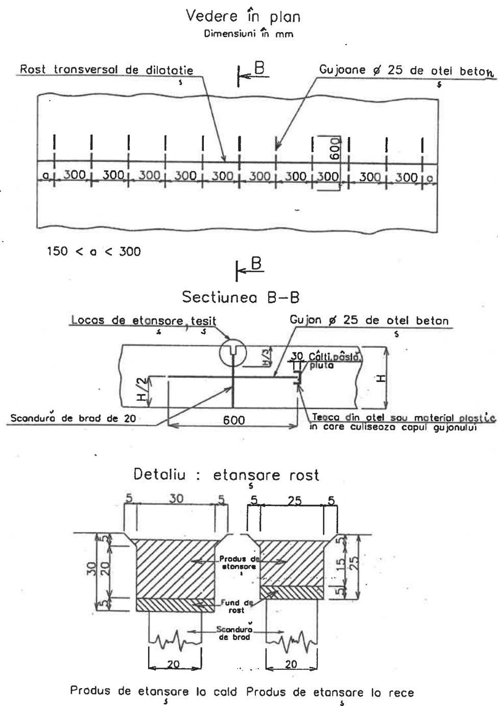
Fig. 21 Rost transversal de dilatație executat cu gujoane
