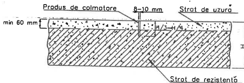
Fig. 16b Rost de contracție transversal, la imbrăcăminti în două straturi, executate cu un singur disc
