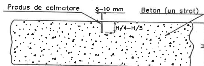
Fig. 15b Rost de contracție transversal, la imbrăcăminti într-un strat, executate cu un singur disc
