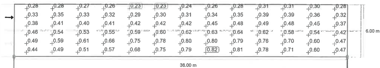
Observator 2: Valoarea de întreținere, densitatea luminii cu carosabil uscat [ \text{cd/m}^2 ] (Linii Isolux)
