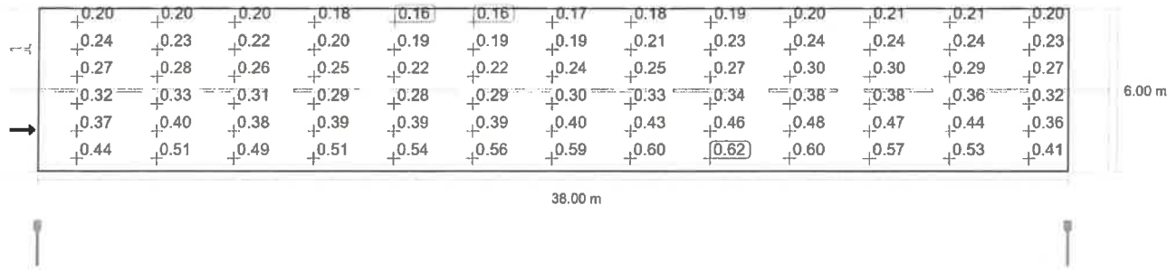
Observator 1: Valoarea de întreținere, densitatea luminii cu carosabil uscat [cd/m²] (Raster valoric)
